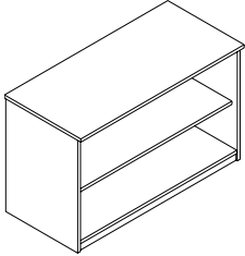
ED650J L367/H650/W492
